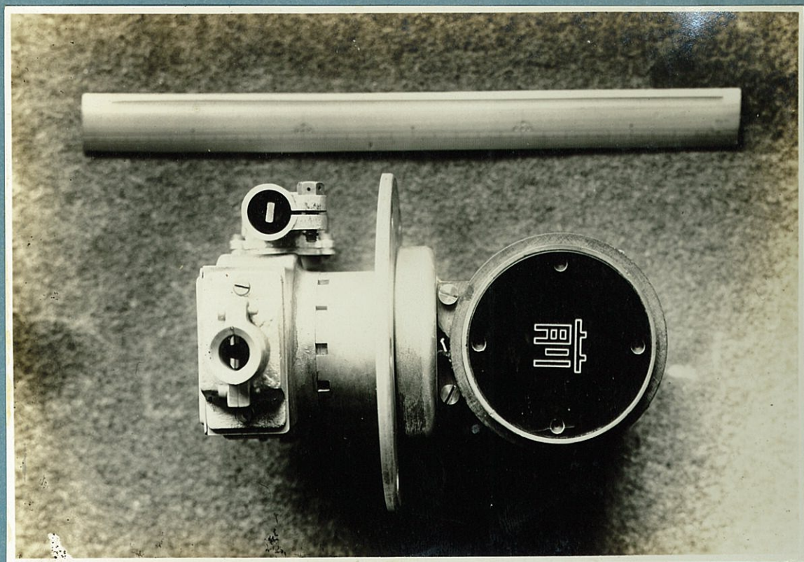
寫 眞 1 5 方 向 探 知 器 ( 其 ノ 一 )
